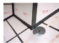
ベージュ部分は外断熱材、黒い部分は気密テープ
